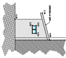
PROSPETTO SUD BASSO FABBRICATO
